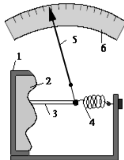
Fig. 3.10. Barometer–Aneroid:
