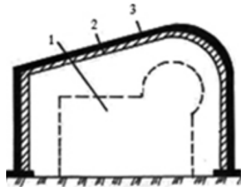
Fig. 8.5. Soundproof Shield:
