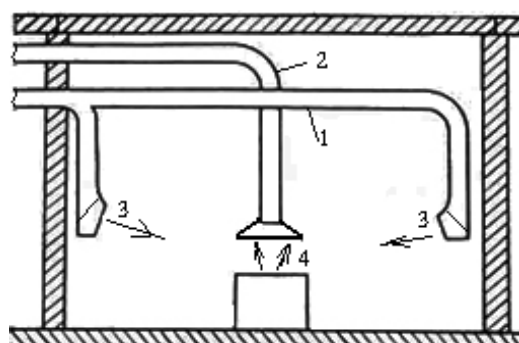
Fig. 4.12. Local Ventilation Scheme:
