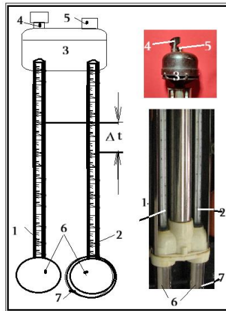
Fig. 3.7. Assmann Psychrometer
