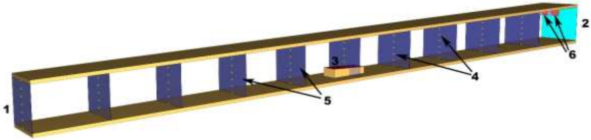
ფიგ. 1.2. ჭავლური ვენტილატორებისა და საზომი მოწყობილობების განლაგება გვირაბის მოდელზე: 1, 2 - ქვედა და ზედა პორტალი, სადაც დამონტაჟებულია ორი, სამი ან ოთხი ცალი ჭავლური ვენტილატორი; 3 - ხანძრის კერა; 4 - წერტილოვანი საზომი მოწყობილობები; 5 - მოცულობითი საზომი მოწყობილობები; 6 - ვენტილატორები დადმავალი სავენტილაციო ნაკადებისათვის
